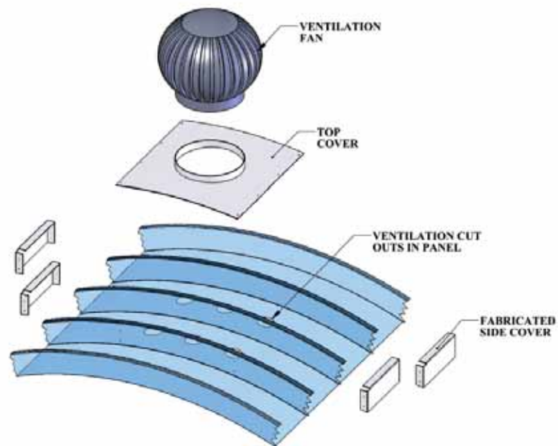
Exhaust Fan Components
